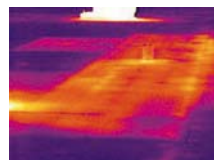
Tetto a terrazzo infiltrazioni d'acqua piovana
